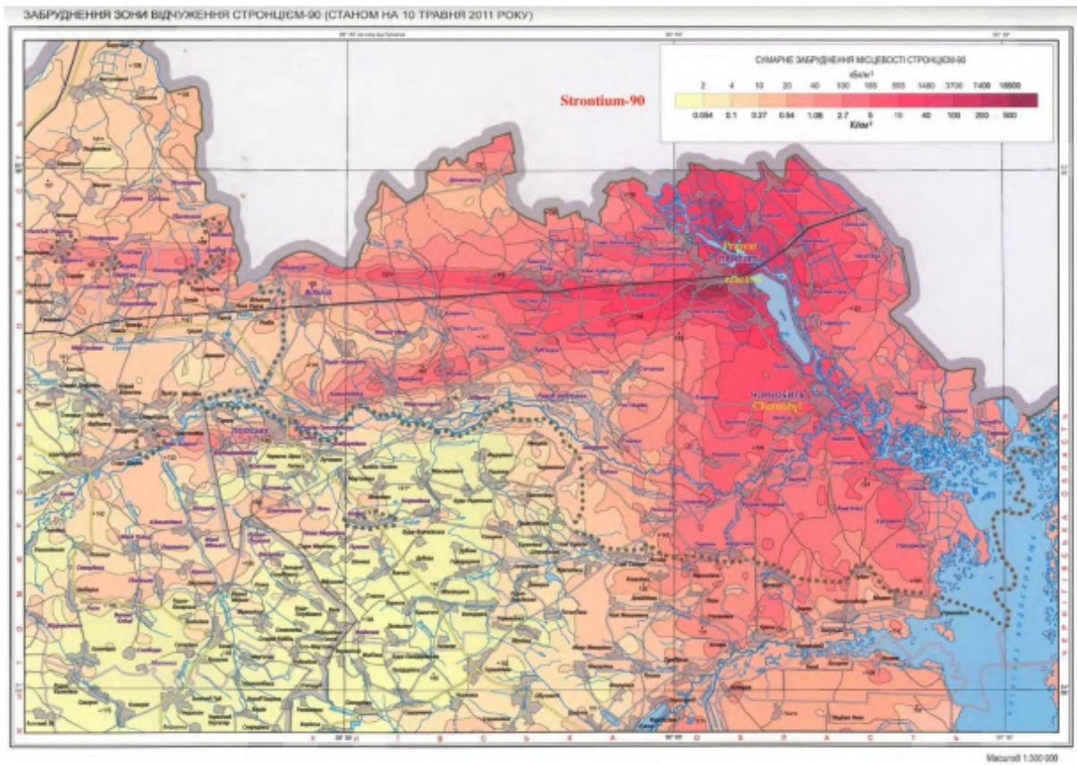
Рисунок А10: Карта осаднения стронция-90 на почве в украинской части зоны отчуждения Чернобыльской АЭС, 2011 г. Верхняя шкала указана в кБк/м 2 , а нижняя шкала в Ки/км 2 .
