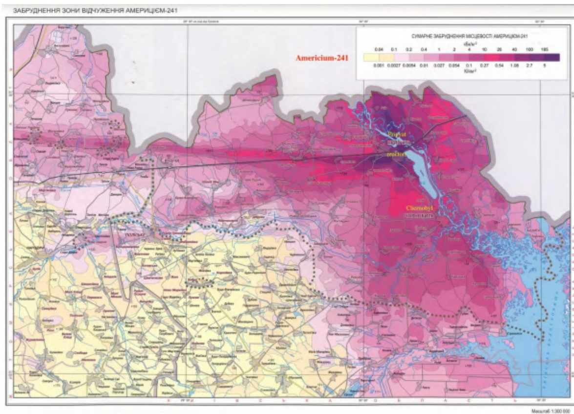
Рисунок А12: Карта осаждения америция-241 на почве в украинской части зоны отчуждения Чернобыльской АЭС, 2011 г. Верхняя шкала указана в \text{kBq}/\text{m}^2 , а нижняя шкала в \text{Ki}/\text{km}^2 .
