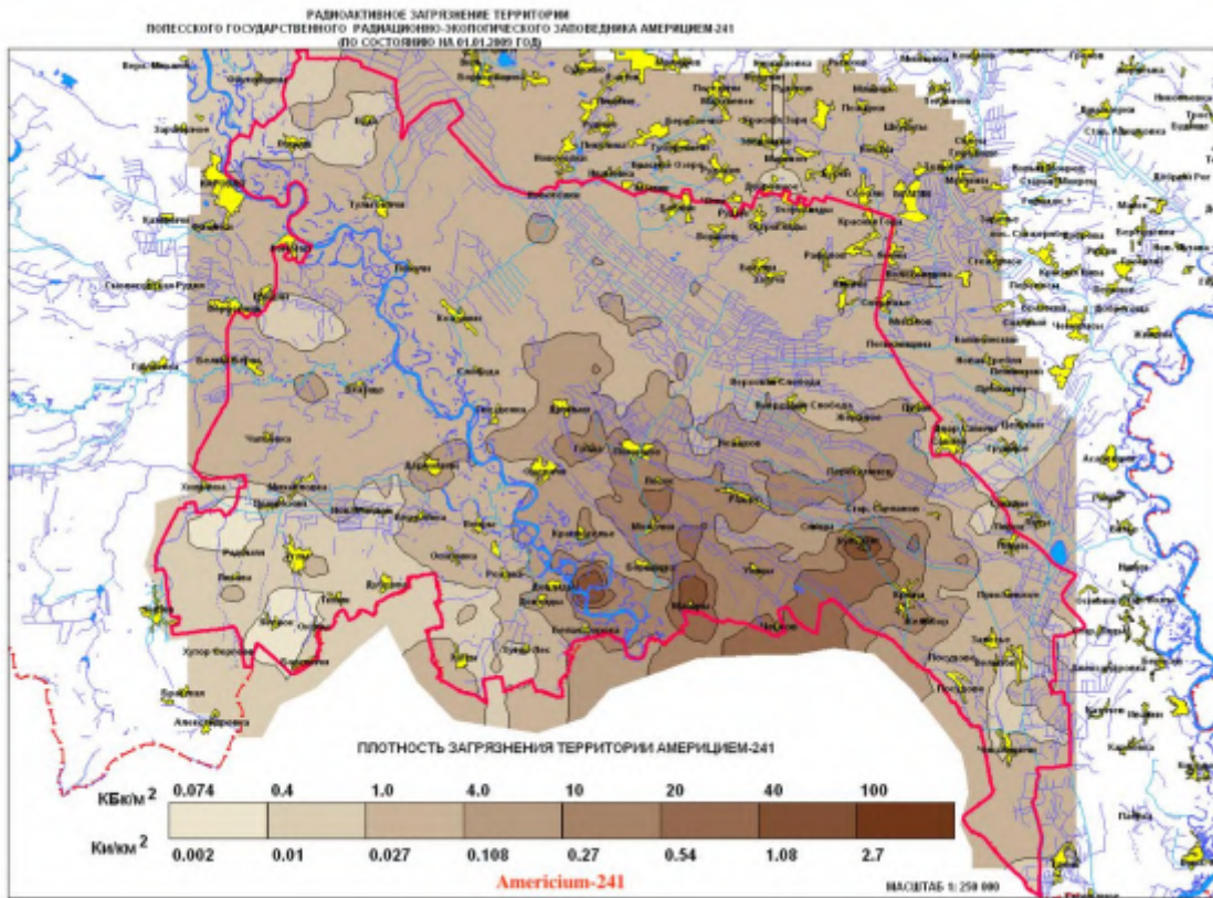
Рисунок А5: Карта 2009 г. осадения америция-241 на почве в белорусской части зоны отчуждения Чернобыльской АЭС. Верхняя шкала указана в \text{кБк}/\text{м}^2 , а нижняя шкала в \text{Ки}/\text{км}^2 .
