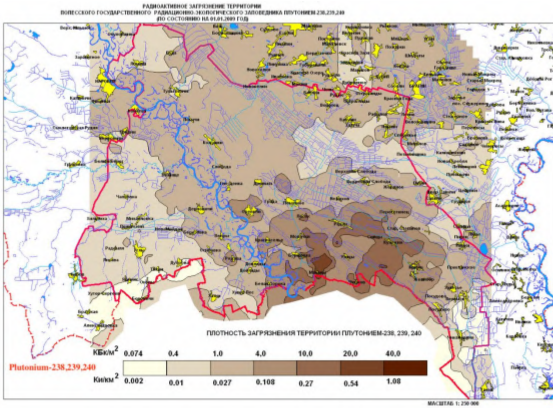
Рисунок А3: Карта 2009 г. осаждения плутония-238, 239, 240 на почве в белорусской части зоны отчуждения Чернобыльской АЭС. Верхняя шкала указана в \text{кБк}/\text{м}^2 , а нижняя шкала в \text{Ки}/\text{км}^2 .
