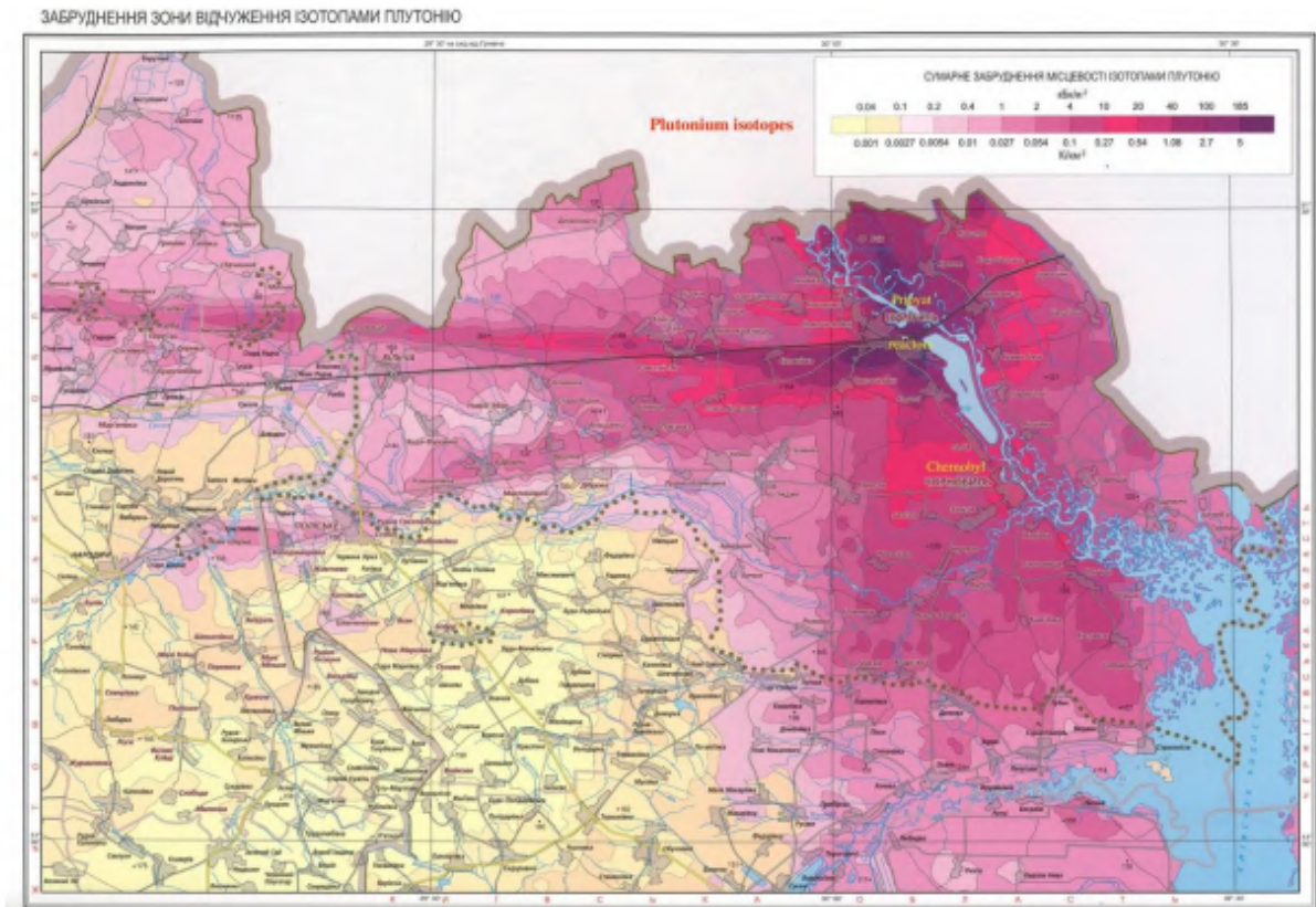
Рисунок А11: Карта осадження ізотопів плутонія на ґрунті в українській частині зони відчуження Чернобыльської АЕС, 2011 г. Верхня шкала вказана в кБк/м 2 , а нижня шкала в Ки/км 2 .
