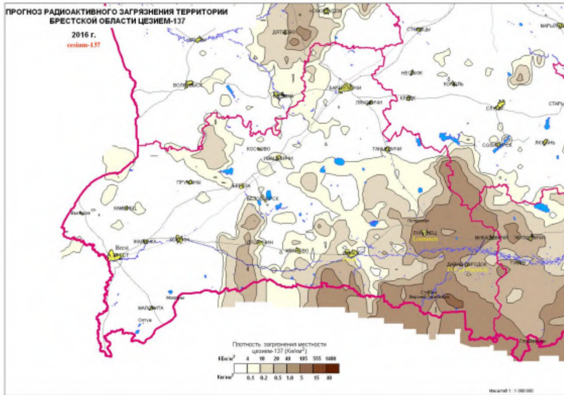
Рисунок А7: Карта 2016 г. осадения цезия-137 на почве в Брестской области. Верхняя шкала указана в kBq/m 2 , а нижняя шкала в Ci/km 2 .
